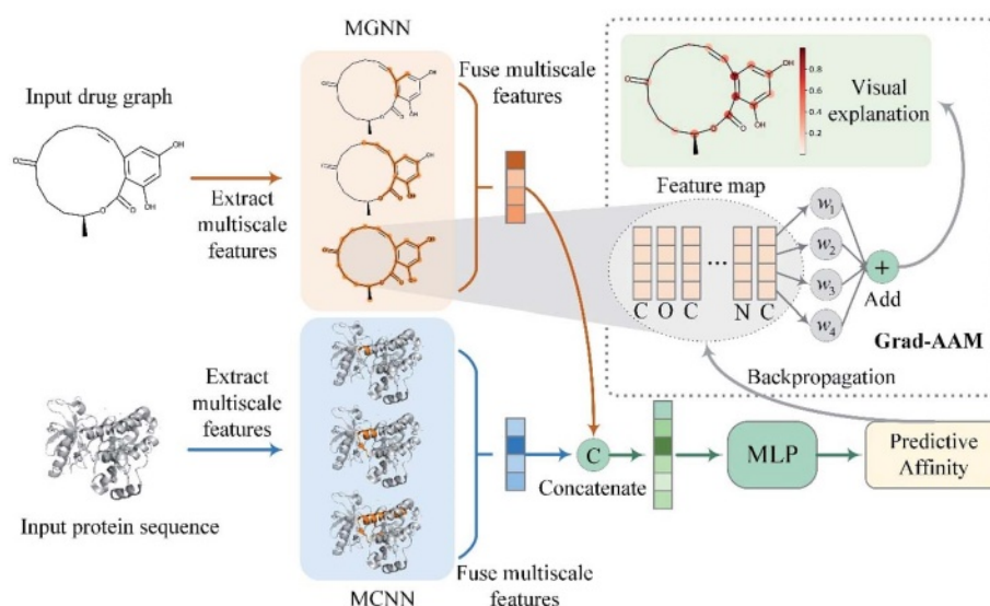
图 2 展示了所提出的 MGraphDTA 模型的概况。MGNN 和 MCNN 分别用于提取输入药物图和蛋白质序列的多尺度特征。将两个编码器输出的多尺度特征分别融合, 然后拼接, 以获得药物-靶点对的组合表示。最后, 将组合表示输入到多层感知机 (MLP) 中以预测结合亲和力。Grad-AAM 利用流入 MGNN 最后一个图卷积层的梯度信息来理解每个神经元对于亲和力决策的重要性。
